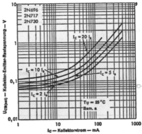
Kollektor-Emitter-Restspannung als Funktion des Kollektorstromes
