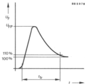
Fig. 1 Einschalt-Überspannungsspitze
