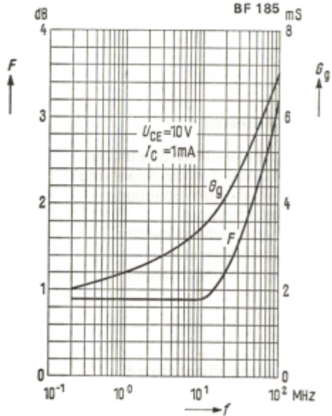
Frequenzabhängigkeit des Rauschens F = f(f) bei optimaler Anpassung U_{CE} = 10\text{ V}; I_C = 1\text{ mA}; T_u = 25^\circ\text{C}
