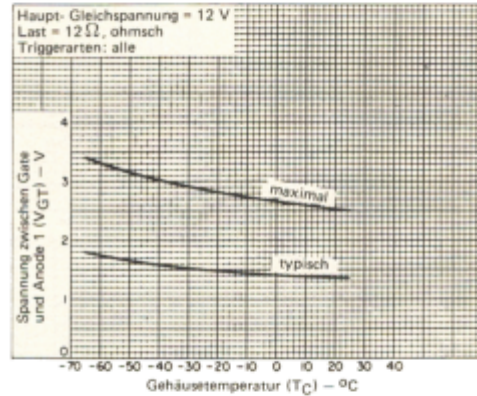
Bild 10: Gate-Triggergleichspannung in Abhängigkeit von der Gehäusetemperatur
