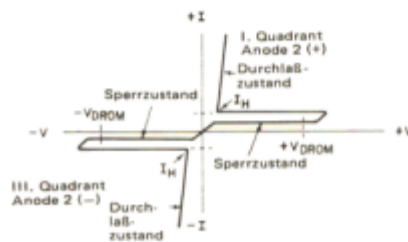
Bild 1 – Strom/Spannungs-Kennlinie (Prinzipdarstellung)
